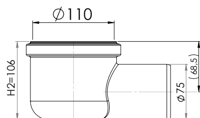
Side Ø75
