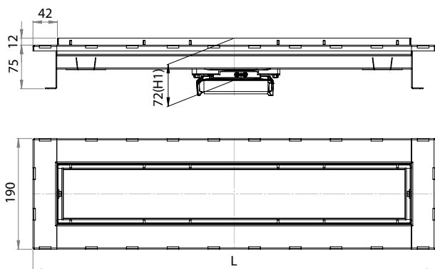
Renne med sentrert utløp, uten fall
