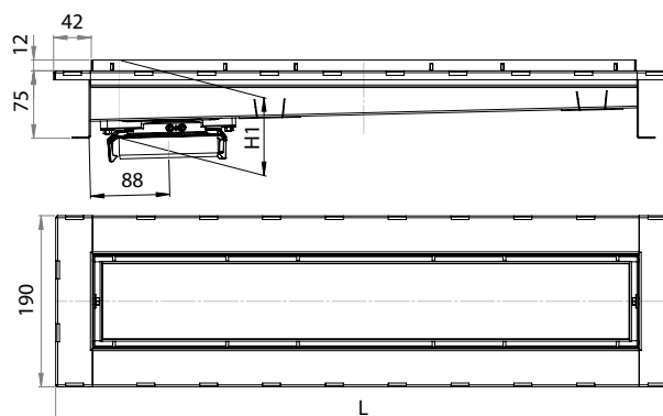
Renne med gavelutløp, med fall (se tabell)
